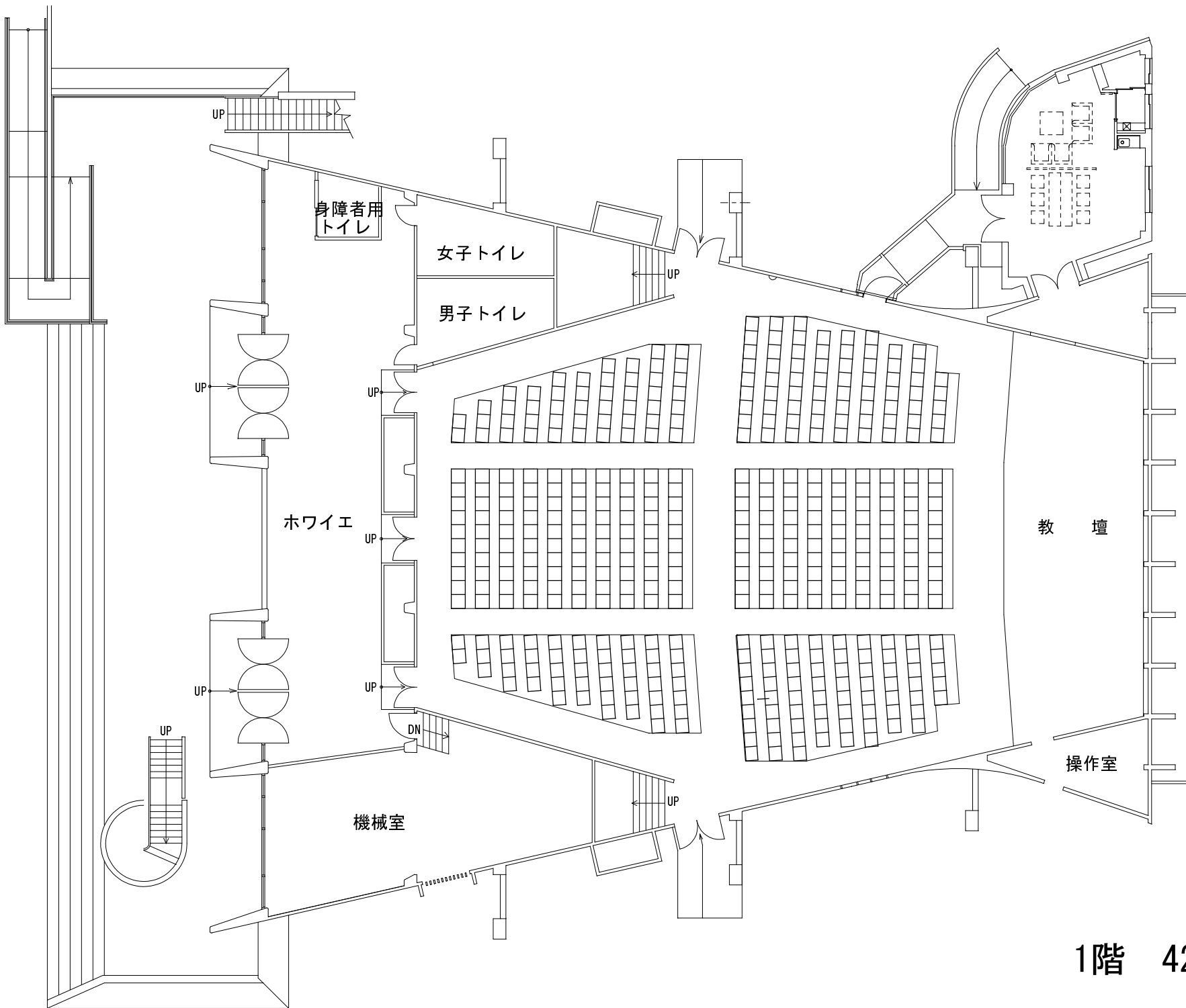
中部講堂 1階平面図
