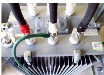
医学部基礎研究棟の高効率変圧器
