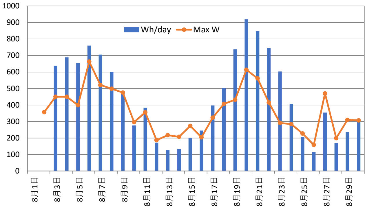
1日の発電量(Wh/day)と最大発電量(W)
