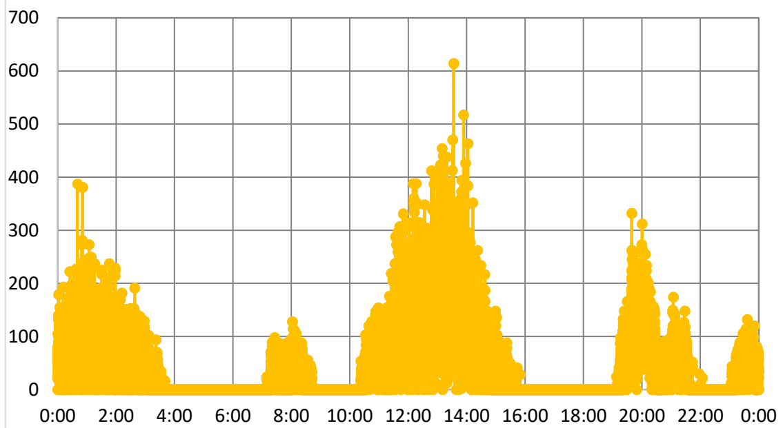
2020年8月20日の発電記録 (1日2回の上潮、下潮において流速が一定値を超える時に発電する)
