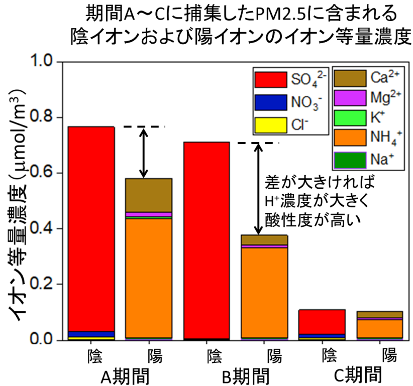
図5 図1の期間A(7月1日)、期間B(7月4日)、期間C(7月5日)に長崎大学文教キャンパスで捕集したPM2.5に含まれる主要な陰イオンおよび陽イオンのイオン等量濃度(イオンの総電荷数)
