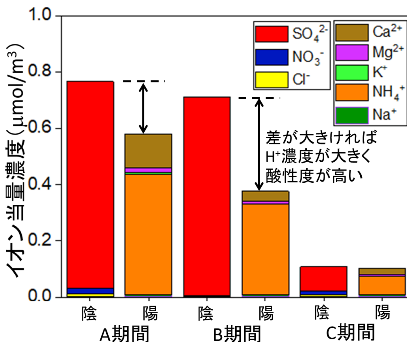
図5 図1の期間A(7月1日)、期間B(7月4日)、期間C(7月5日)に長崎大学文教キャンパスで捕集したPM2.5に含まれる主要な陰イオンおよび陽イオンのイオン当量濃度(イオンの総電荷数)
