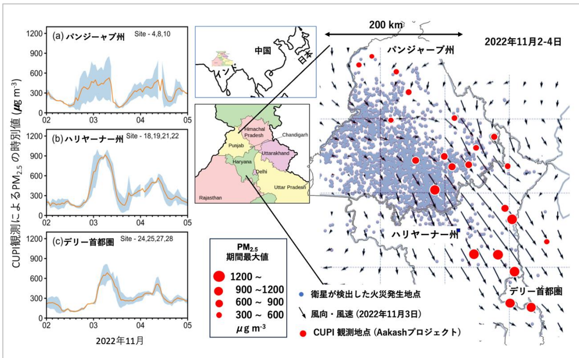
図1：2022年11月2-4日の農業残渣物燃焼によるパンジャブ州におけるPM 2.5 の放出とデリー首都圏への輸送の事例。赤丸が観測点の位置を示す。左図ではパンジャブ州、ハリヤーナー州、デリー首都圏におけるPM 2.5 濃度の変化（オレンジと水色はそれぞれ同一州内複数地点の時間平均値と標準偏差を意味する）、右図では本期間における
