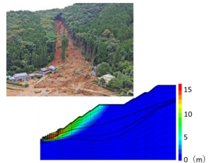
【図-1】斜面地盤の数値シミュレーション
