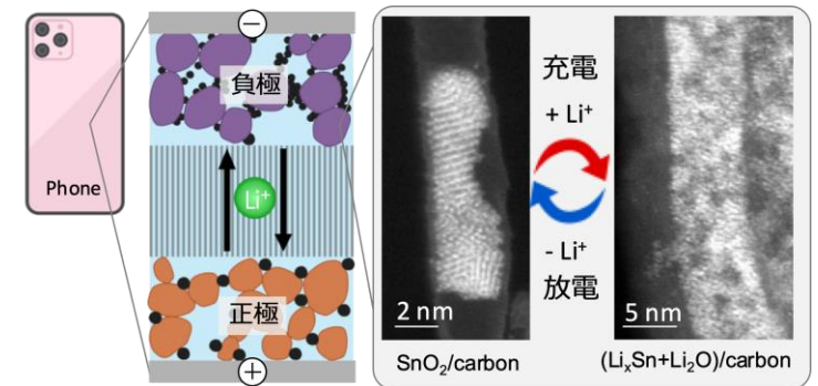
リチウムイオン電池の模式図と充電、放電後の電極活物質(SnO 2 /カーボンナノチューブ複合体)の電子顕微鏡像
