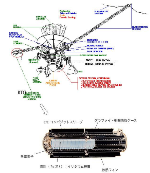
(右図は、NASA 惑星探査宇宙船ガリレオに搭載された RTG(放射線同位元素を使った熱電発電器)。(KOMATSU のHPより))
